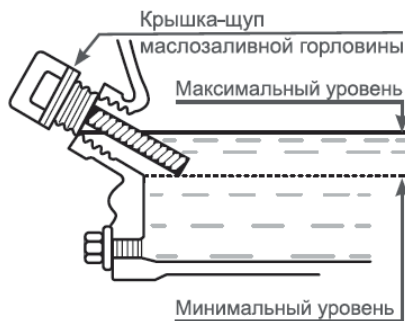
Проверка уровня масла в картере
