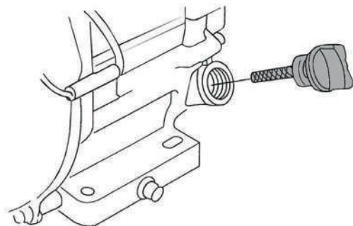
Крышка-щуп маслозаливной горловины
