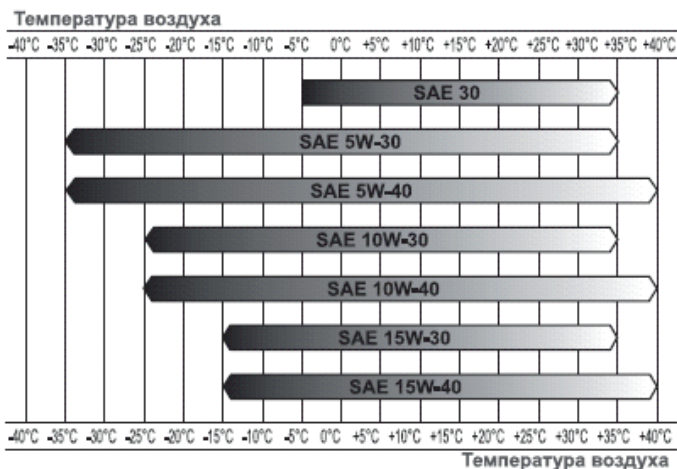
Рис. 10 Определение вязкости масла
