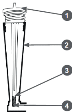
Рис. 12 Уровень масла в картере двигателя 1. Крышка-щуп 2. Горловина маслосазливная 3. Максимальный уровень масла в картере 4. Минимальный уровень масла в картере
